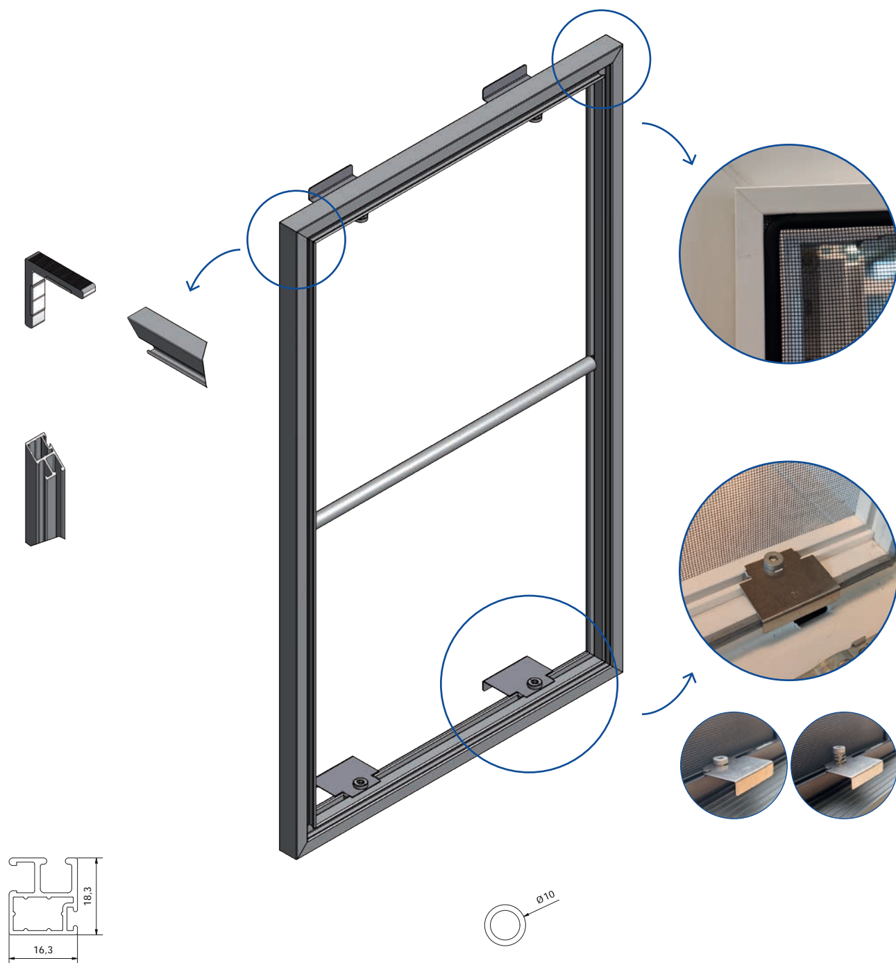
VR050 Dormant 16,3 mm
