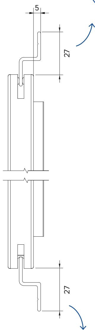
VP1012 Guide inférieur 13,5 mm
