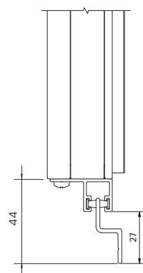
VP1012 Guide inférieur 13,5 mm
