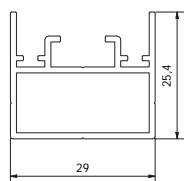
VP4002 Dormant horizontal inférieur
