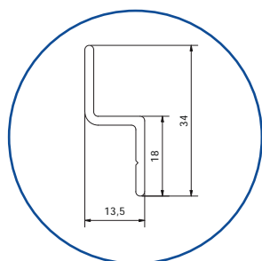
VR073 Guide inférieur 21 mm
