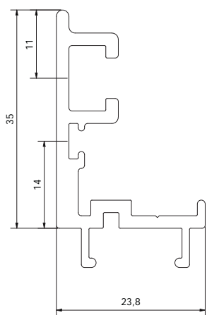
VP1010 Profil de roulement
