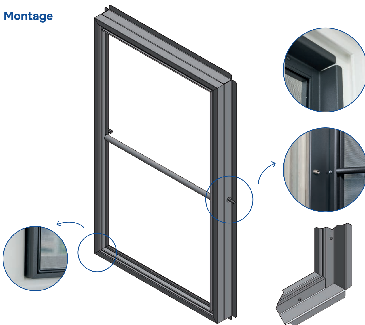
VR050 Dormant 16,3 mm
