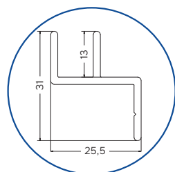
VP1059/VP1060 Guide inférieur 31 mm
