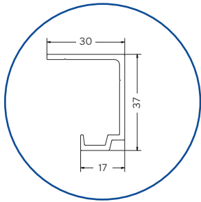
VP5088 Guide supérieur 30 mm
