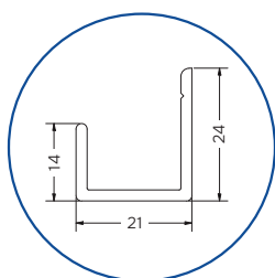
VP1054 Guide inférieur 21 mm
