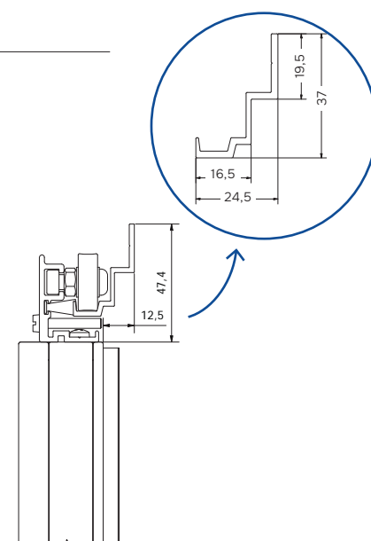
VP1011 Guide supérieur 5 mm
