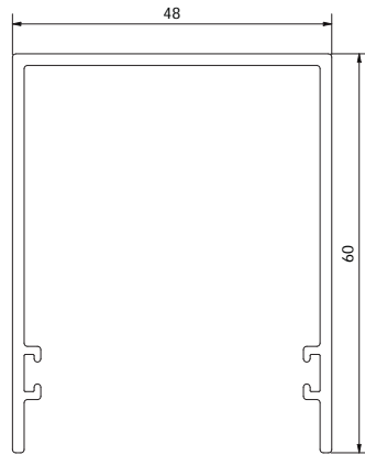
VP4011 Guide supérieur
