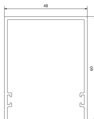
VP4011 Guide supérieur de 1400 mm*
