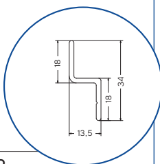
VP1012 Guide inférieur 13,5 mm
