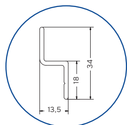
VP1012 Guide inférieur 13,5 mm
