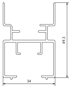
PL0801 Profil coulissant
