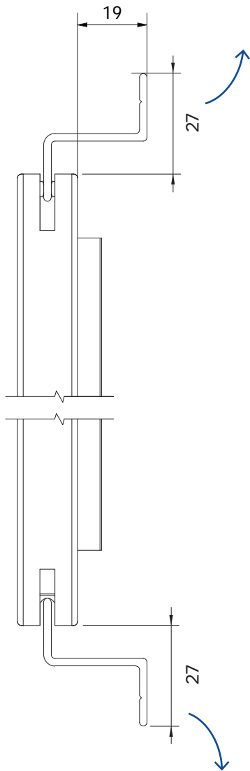
VR074 Guide inférieur 27,5 mm
