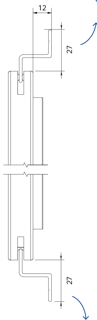
VR073 Guide inférieur 21 mm
