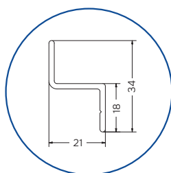
VR073 Guide inférieur 21 mm
