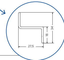
VR074 Guide inférieur 27,5 mm
