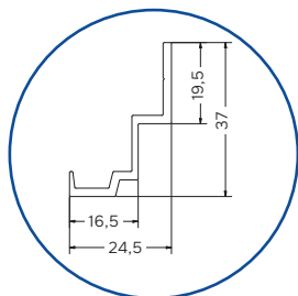
VP5088 Guide supérieur 30 mm
