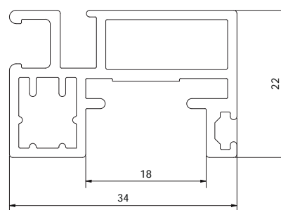
VP1018 Ouvrant pour tôle
