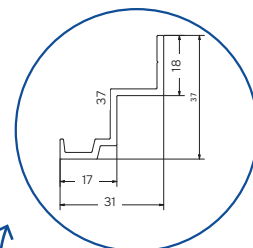
VP4961 Guide supérieur 10 mm
