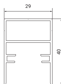
VP4004 Dormant horizontal supérieur
