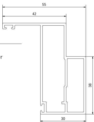
VP1018 Ouvrant pour tôle
