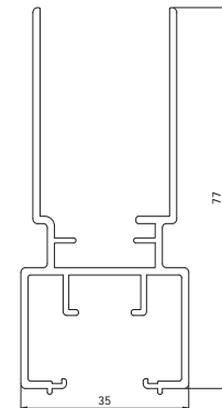
PL0804 Profil fixe 78,4 mm (à partir d'une largeur de 1200 mm)
