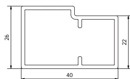
VP1020 Traverse pour tôle
