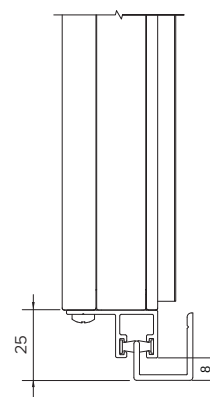
VP1054 Guide inférieur 21 mm
