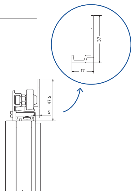
VP5087 Guide supérieur
