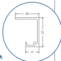
VP5088 Guide supérieur 30 mm
