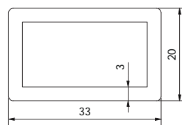
VP1040 Tube rectangulaire ouvrant pour le renforcement à partir de 1800 mm de largeur
