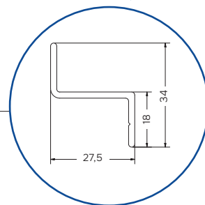
VR074 Guide inférieur 27,5 mm
